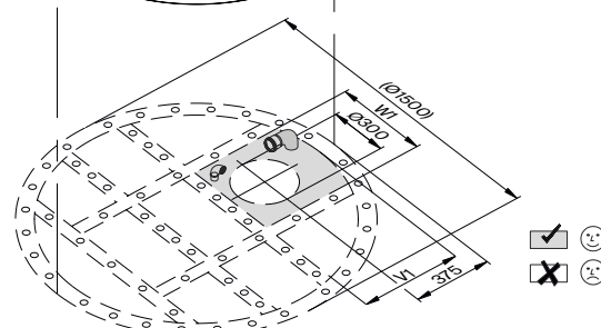
Anschlussmaße für Ab- und Überlaufgarnitur
