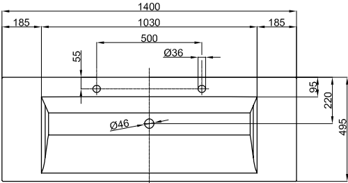
Abb.: BetteAqua 1400 × 495 mm mit 2 Hahnlöchern
