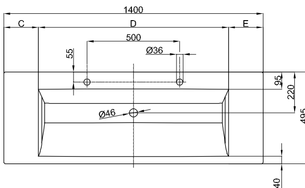
Abb.: BetteAqua 1400 x 495 mm mit 2 Hahnlöchern
