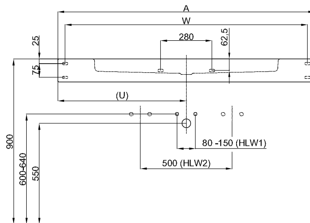
Montage- und Anschlussmaße:
