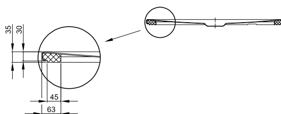
Darstellung mit vormontiertem Minimum-Wannenträger (T1).
