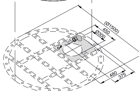
Anschlussmaße für Ab- und Überlaufgarnitur
