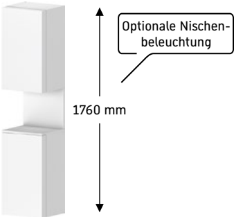
Hochschrank wandhängend, 2 Türen L/R, offene Ablage, Einlegeböden aus Glas im oberen Teil des Schrankes
