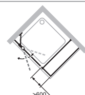
Mit Querverstrebung.
