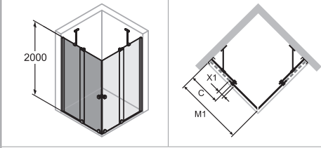
Linksbefestigung
